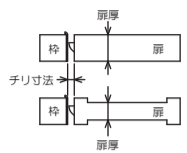
図1-1-1 チリ寸法と扉厚
