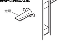
図1-1-2 扉厚の測定方法
